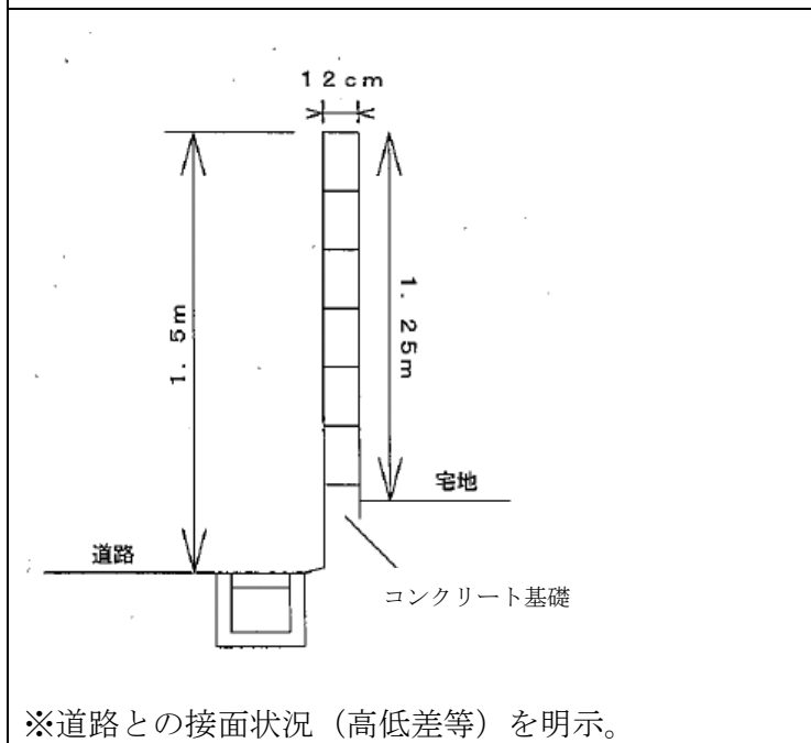
側面図 (その1)
